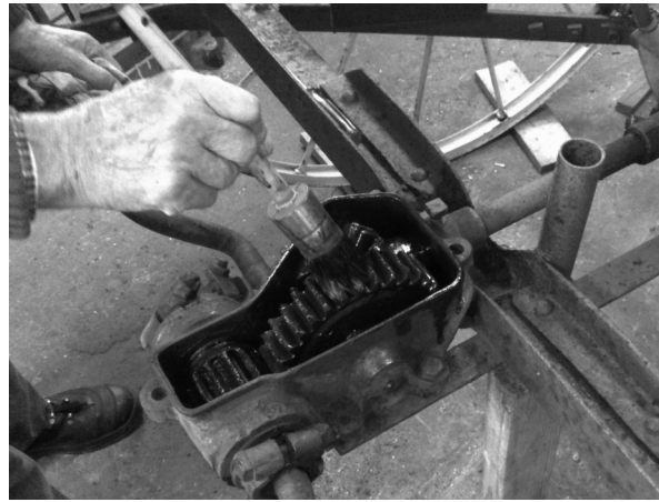
Deel van de mechaniek van een hooidraaier.
