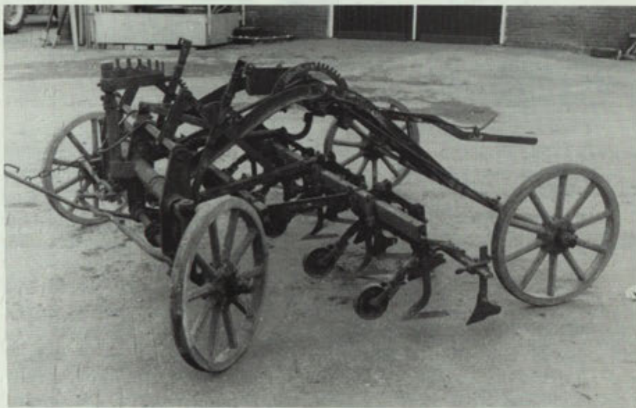
De schoffelmachine
