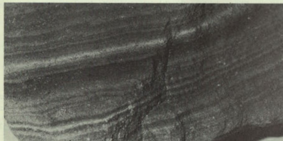
Deze foto laat duidelijk zien dat onze "mergel" een afzettings- of sedimentsgesteente is, gesteente dat uit lagen bestaat.
