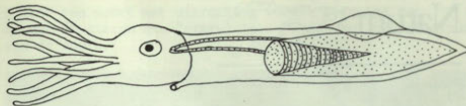
Reconstructie van een belemniet. De harde delen (gestippeld) kunnen we tegenwoordig als fossielen terug vinden. We noemen ze "donderkeilen".
