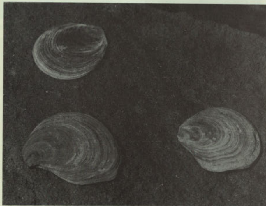
Overblijfselen van schelpdieren uit de Krijttijd, gevonden in de "mergel" bij Rijckholt.
